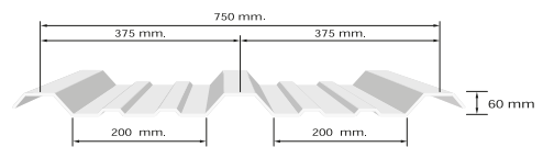
WMI 60-750BL
