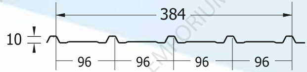
TYPE 5RIB
