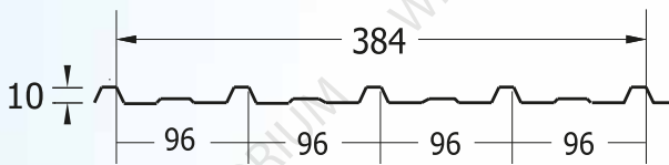
TYPE 5S
